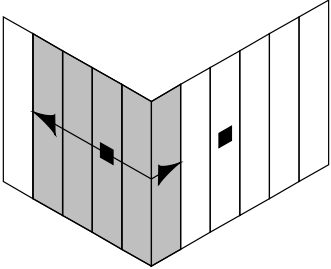
Eckverbindung Wand/Wand durchgehend verschweißt
