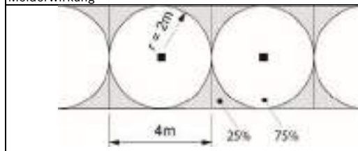
Melderwirkung
