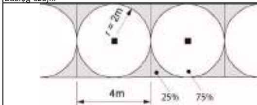
Zasięg czujki
