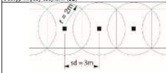
Odstęp między czujkami (sd)
